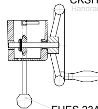
FHES.23A0.00 Schalthebel
