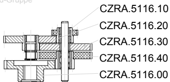
CZRA.5116.___ Zahnrad-Gruppe
