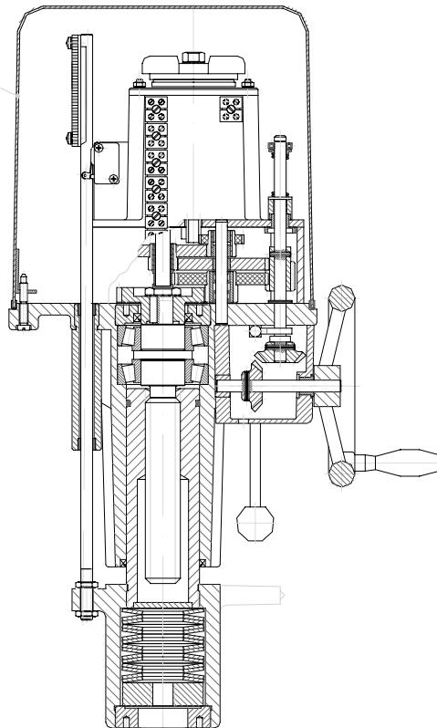
CWEK.5116.00 Kupplungswelle-Gruppe
